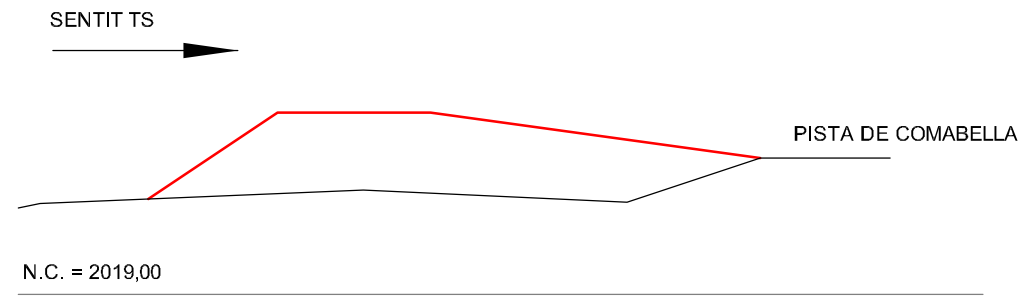
PERFIL A-B
