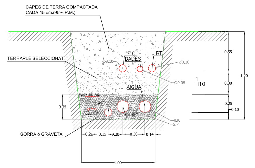
SECCIÓ TRANSVERSAL ESCALA 1:50
